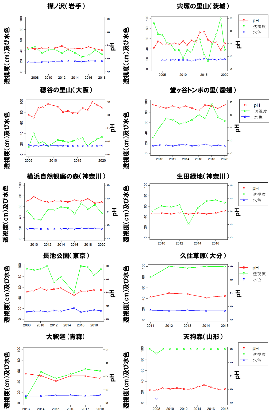
図 3-12 各地の調査サイトの止水域（溜池や沼）での水質の変化。
