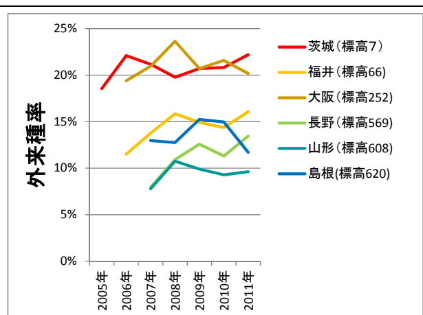
図 2-29: 調査を 5 年以上しているサイトにおける外来種率の経年変化。凡例の括弧内の数字はそのサイトの標高(m)を現す。
