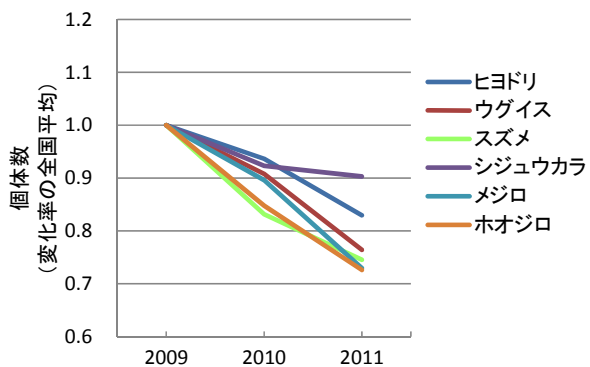
図 2-5: 優占度の高い主要な留鳥6種の記録個体数の全国平均。各サイトでの記録個体数の相対変化(初年度を1とした変化率)を求め、それを相乗平均した。
