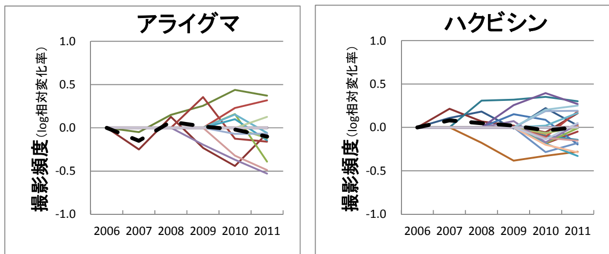
図 2-31: アライグマ(左)及びハクビシン(右)についての各調査サイトでの撮影頻度の経年変化。縦軸は初年度を1とした時の相対変化率を対数変換した値を示しているため、初期値は0となっている。カラーの折れ線は各サイトの変化、黒色の点線はその全国平均を表す。
