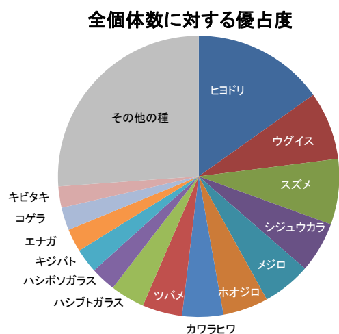
図 2-4: 全記録個体数に占めるそれぞれの種の優占度の全国平均。それぞれのサイトについて、種ごとの優占度(全個体数に占める個体数の比率)の過去3年の平均を算出し、それを全サイトで平均して求めた。
