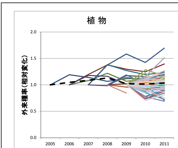
図 3-28: 植物の外来種率(全種数に占める外来種の比率)についての全国的な推移。各サイトの調査初年度の値を 1 とした相対変化として表した。
