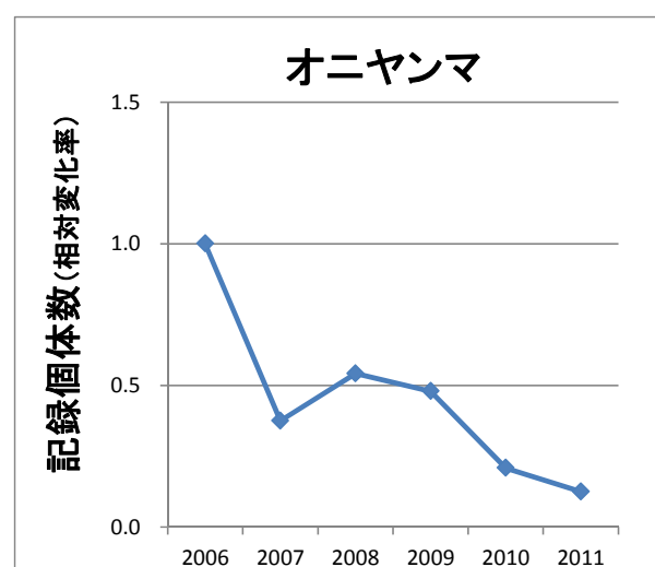
図 2-15: 大阪のコアサイトにおけるオニヤンマの記録個体数の経年変化。数値は初年度を1とした時の相対値。
