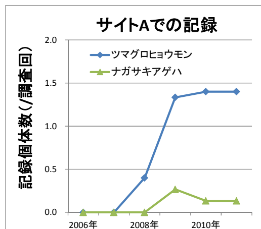
図 2-23: 関東地方にあるサイト A における南方系チョウ類 2 種の記録個体数の経年変化。
