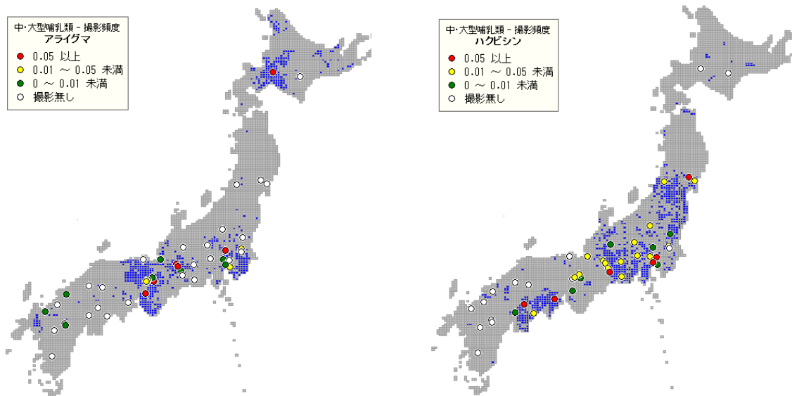
図 2-30: 2011 年の調査におけるアライグマ(左)及びハクビシン(右)の全国での撮影状況。丸の色は撮影頻度(個体/日)の違いを表す(白:撮影無し、緑:0.01 未満、黄:0.01~0.05 未満、赤:0.05 以上)。背景の青色は過去(アライグマ: 2008 年、ハクビシン: 2002 年)の調査での分布地域を表す。
