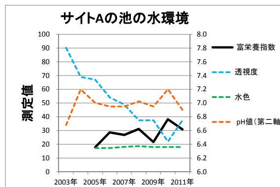
図2-21: 富栄養化指数の増加傾向が確認されたサイトAの溜池における各測定値の経年変化。関東の平野部に位置するサイトで、溜池は水深2mほどと浅く、50haほどの集水域には二次林や畑地が含まれる。
