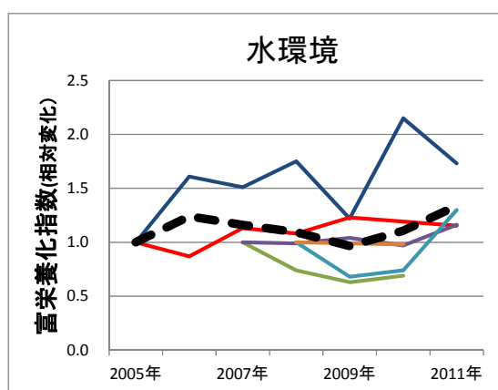
図2-20: 全国のサイトの止水域(溜池や沼)での富栄養化指数の推移。カラーの折れ線は各サイトの最も代表的な止水域での測定結果の相対変化を表し、点線はその全国平均を表す。
